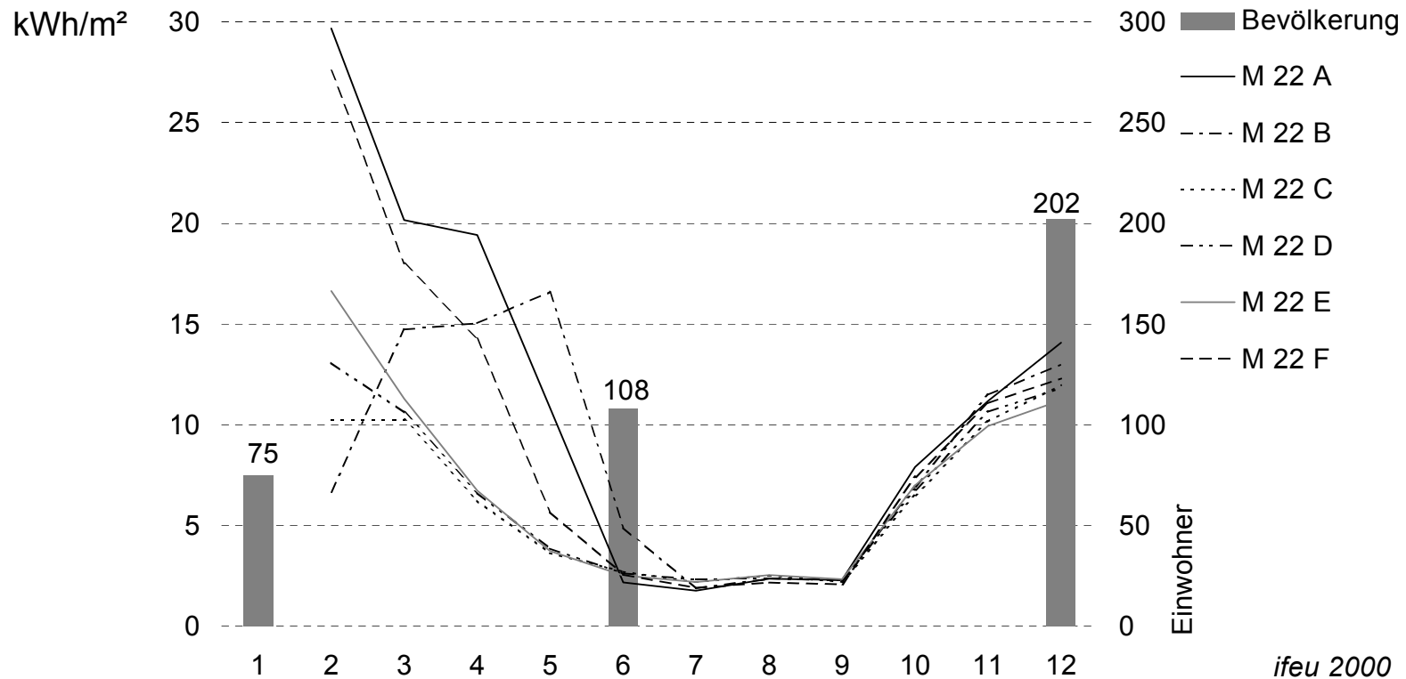
monatlicher Wärmeenergieverbrauch 1999 im Baufeld M 22 bezogen auf die Energiebezugsfläche
