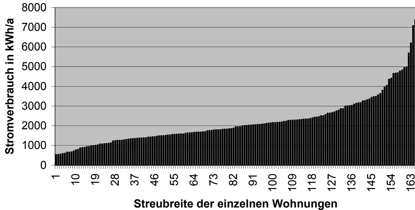
Jahresstromverbräuche Hannover Kronsberg
